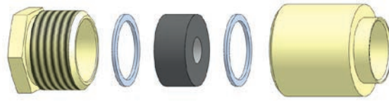
Ausrüstungsart „W“ für Kabel mit Schirmung
