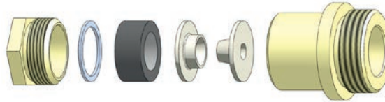
Ausrüstungsart „Z“ für Kabel mit Schirmung
